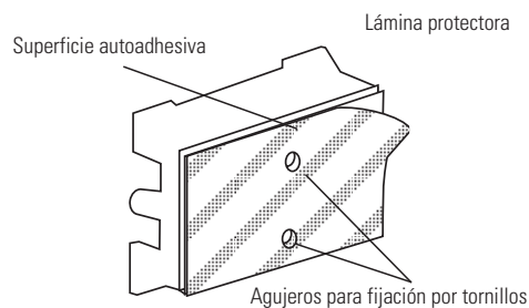
Agujeros para fijación por tornillos
